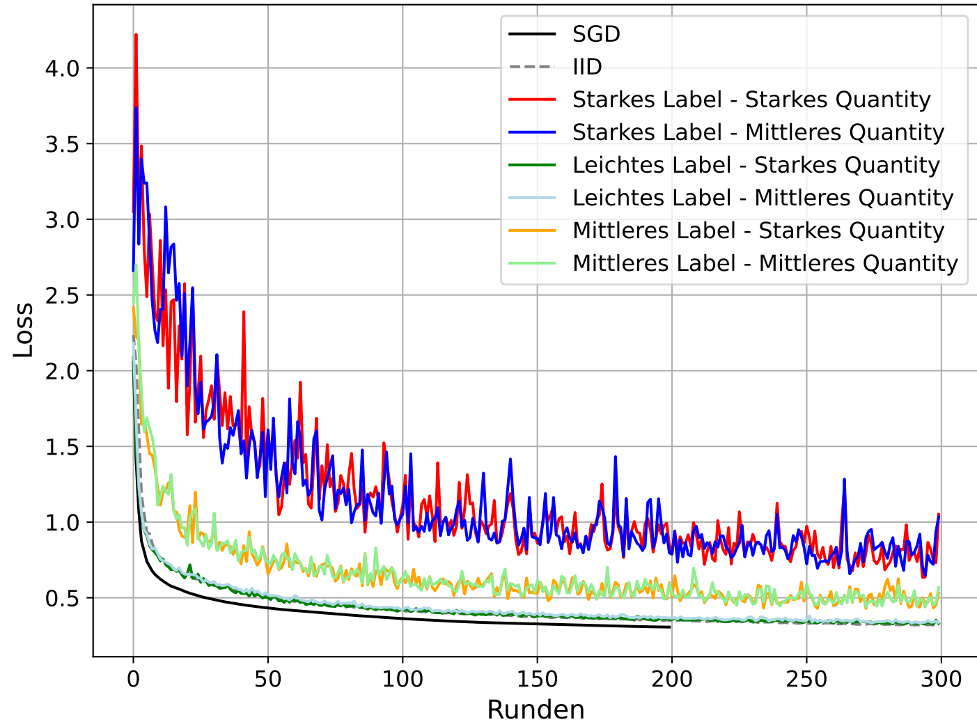
Label Skew & Quantity Skew kombiniert Loss
